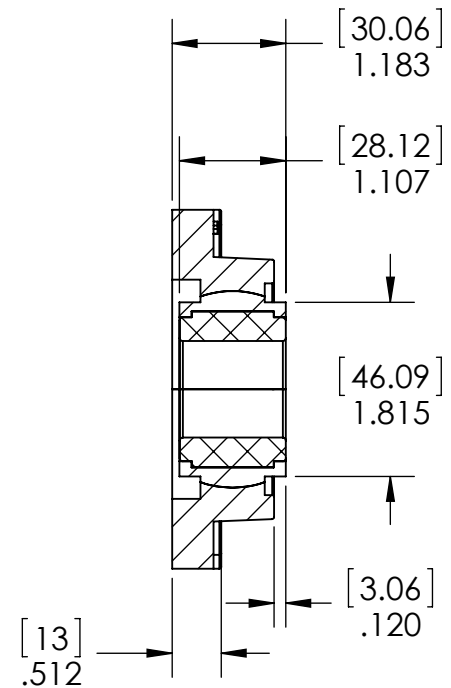
SECTION T-T SCALE 1 : 2
